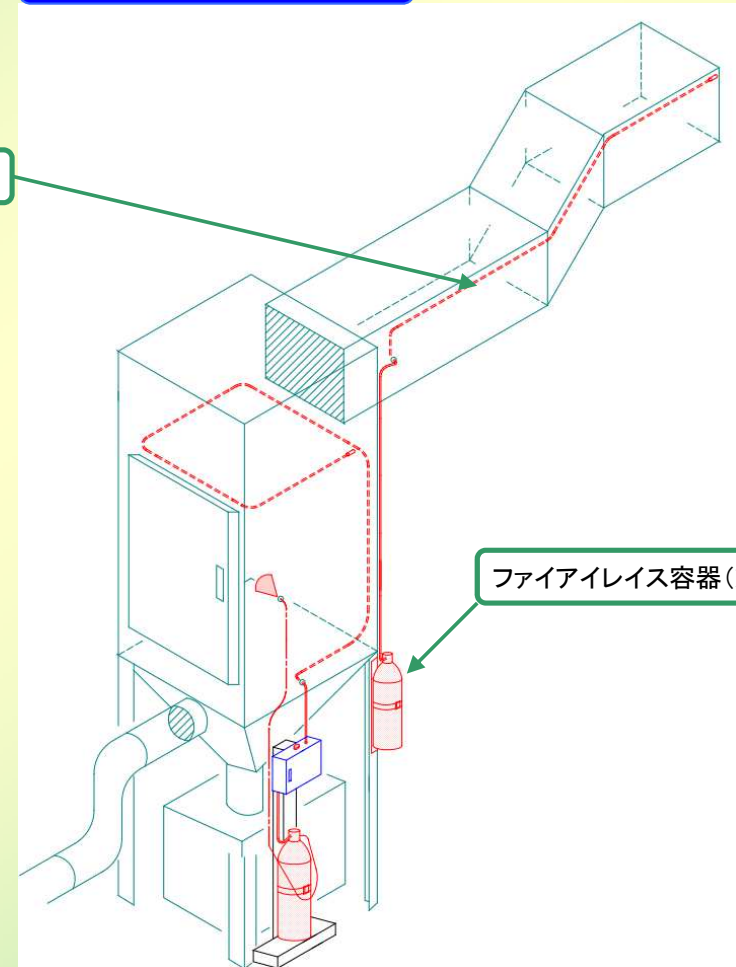
集塵機
